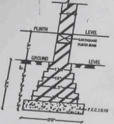
FOUNDATION DETAIL (N.L.S)
